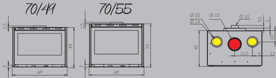
@ Régulateur de la ventilation forcée (V) @ Regeleenheid van geforceerde ventilatie (V) @ Kontrolleinheit des Warmluftgebläse (V) @ Forced ventilation control unit (V)
